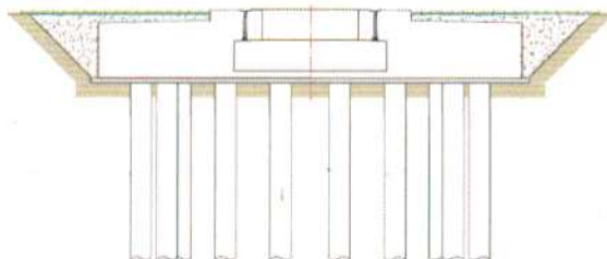
Figura 9 Schema fondazione
