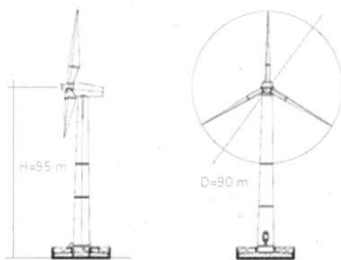
Figura 8 Schema aerogeneratore
